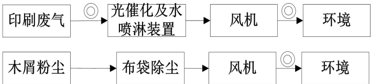
图4-3 废气处理设施流程图
