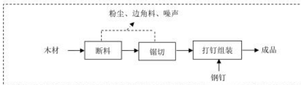
图 3-4 木托生产工艺流程图
