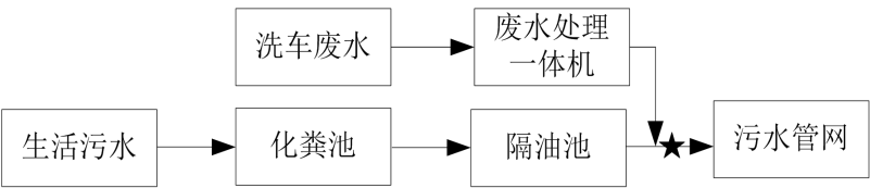
图4-1 废水处理流程图
