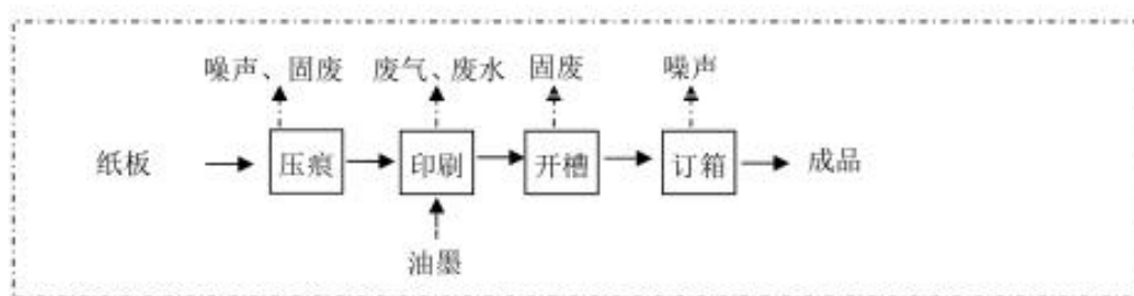
图 3-3 纸制品包装印刷品生产工艺流程图
